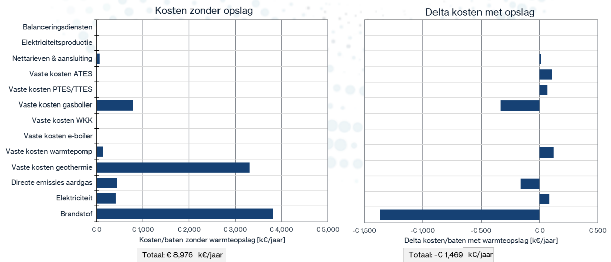
Figuur 6: Uitsplitsing van kosten en baten zonder warmteopslag (links) en de kosten en baten delta met warmteopslag (rechts) (HT-ATES + TTES 3000 m 3 ) voor casus 1.
