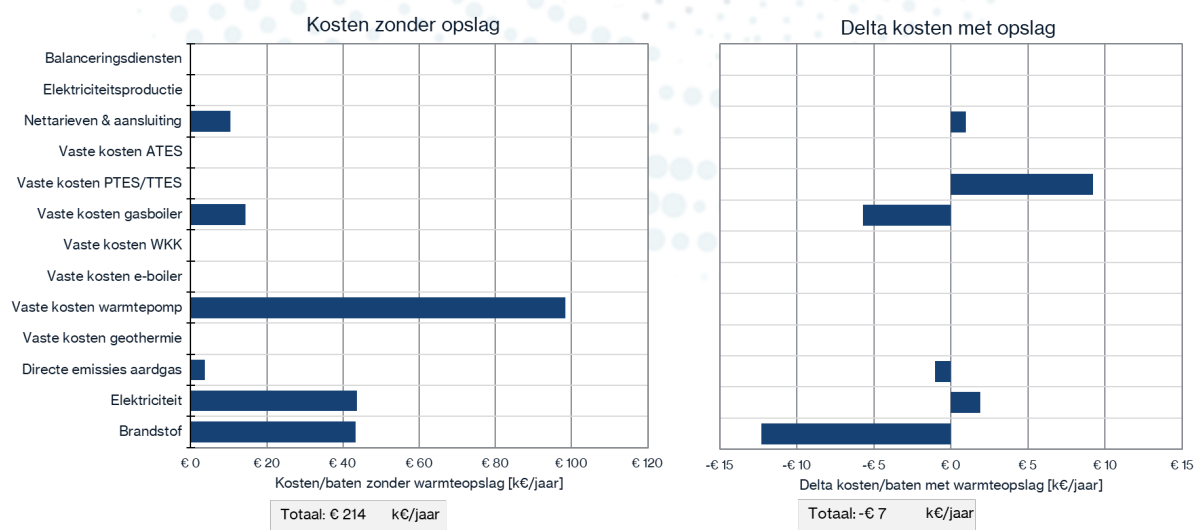
Figuur 18. Uitsplitsing van kosten en baten zonder warmteopslag (links) en de kosten en baten delta met warmteopslag (rechts) (PTES 250 m 3 ) voor casus 3.
