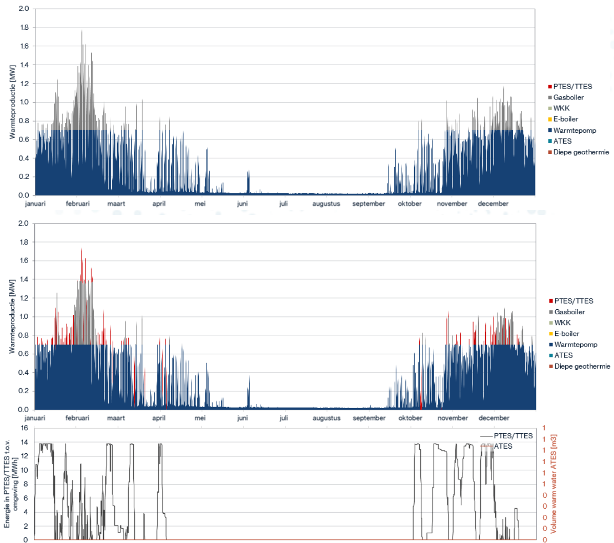
Figuur 20: Uurlijkse inzet warmteproductiemiddelen zonder (boven) en met (onder) warmteopslag (PTES 250 m 3 ) voor casus 3.
