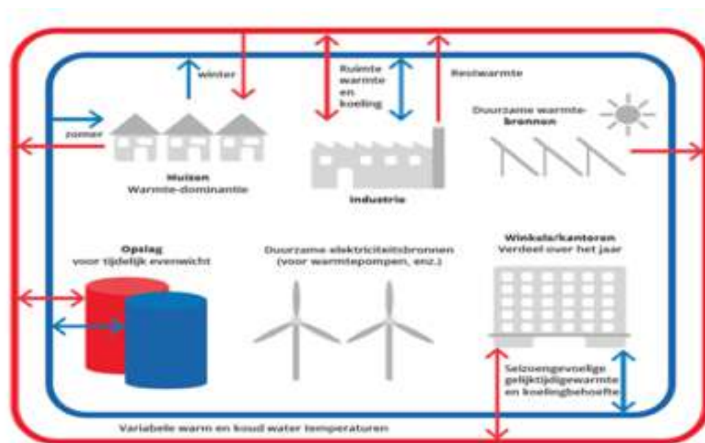
Figuur 4.3.1 5GDHC (5e generatie warmte- en koudenet) 59
