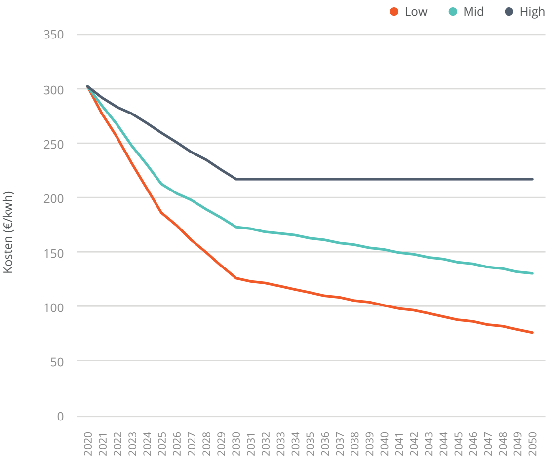
Figuur 8 Initiële kosten van een volledig 4-uur-batterijsysteem. 10
