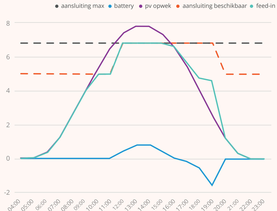
Figuur 24 Benutting van aansluitingscapaciteit wanneer de batterij voor FCR en peakshaving wordt gebruikt op een zonnige lentedag. 21
