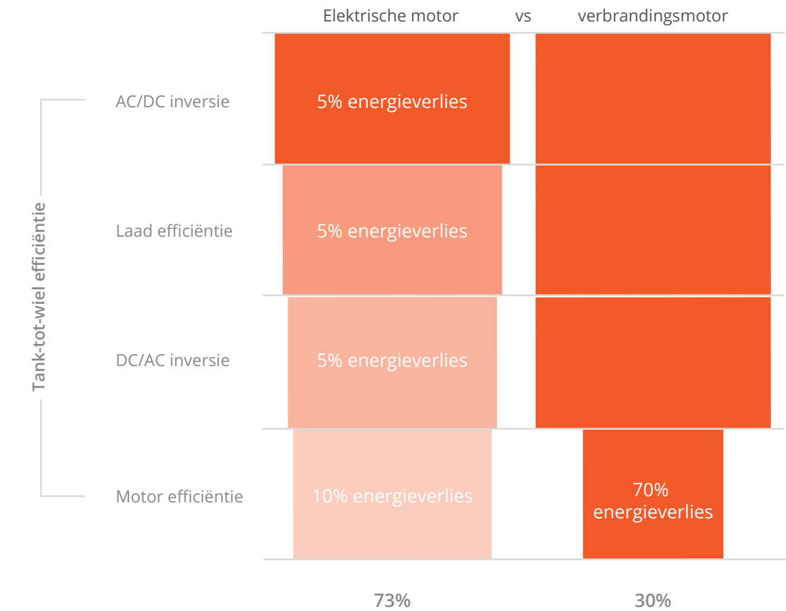
Figuur 32 Tank-to-wheel efficiëntie van een verbrandingsmotor en elektrische motor. 32
