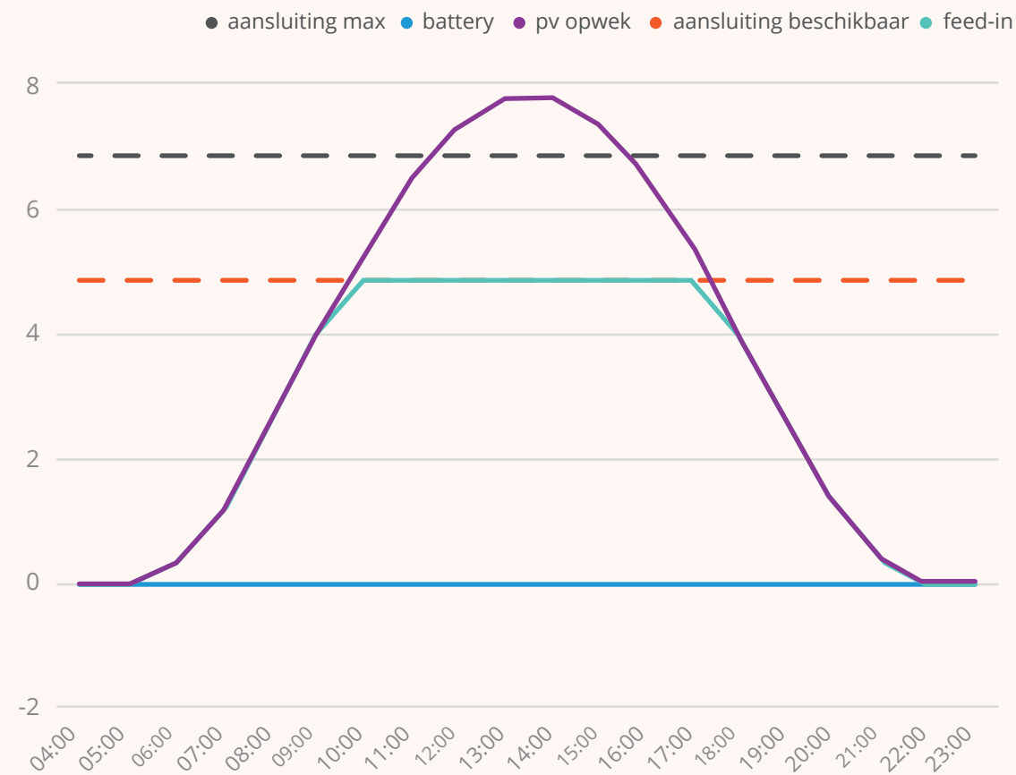
Figuur 23 Benutting van aansluitingscapaciteit wanneer de batterij alleen voor FCR wordt op een zonnig lentedag. 21
